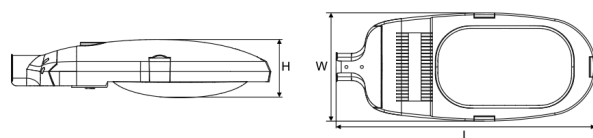
外形寸法：（単位：mm）
