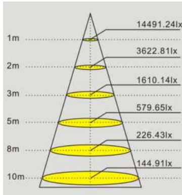
ST-T400100 (配光角60度)
