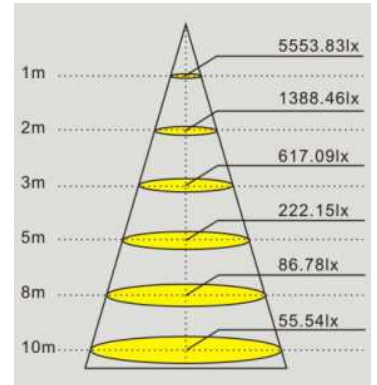
ST-T400100 (配光角120度)
