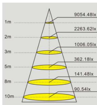
ST-T400100 (配光角90度)
