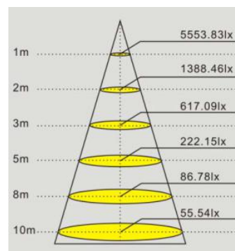
ST-T400100 (配光角120度)
